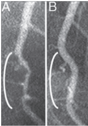
Abb.o.2 Die beiden Röntgenbilder zeigen einen Abschnitt der linken Herzkranzarterie, die einen Großteil des Herzens mit Blut versorgt. Links (A) sieht man das erkrankte Gefäß (der weiße »Schlauch«, der wie ein Ast aussieht und von oben nach unten verläuft – beachten Sie die Verengung im Bereich der weißen Klammer, als wäre der Schlauch zusammengedrückt, was den Blutfluss bremst). Das rechte Bild (B) zeigt dasselbe Gefäß nach 32 Monaten einer in diesem Fall streng veganen Diät, bei der man sich ausschließlich von Pflanzen ernährt. Die Verengung
