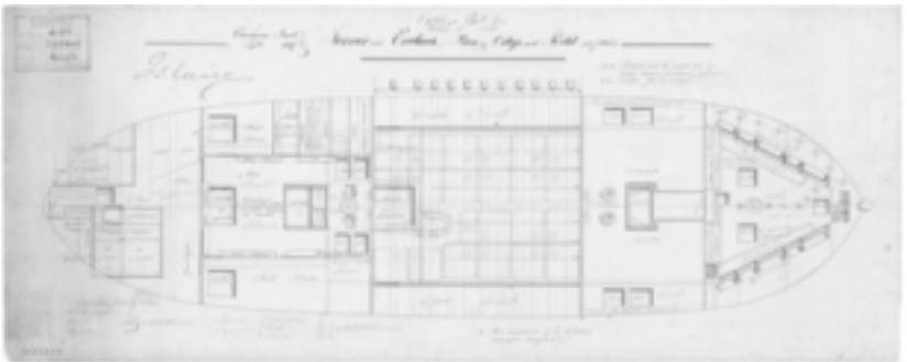
Zwei zeitgenössische Pläne zeigen die Seitenansicht einer typischen Bombarde (oben) sowie das Orlopdeck und die Lagerräume der Erebus und ihres Schwesterschiffes Terror (unten).
